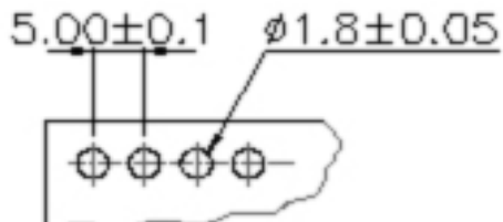
P.C.B HOLDER
