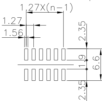
P.C.B LAY OUT
